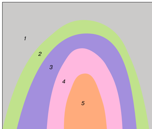
Рис. 2. Схематическое строение гранитогнейсового купола в Шарыжалгайском комплексе, Юго-Западное Прибайкалье (по Е.Б. Курдюкову): 1 — кристаллосланцы ( Orx + Cpx + Hbl + Pl + Bt + Qtz ); 2 — гнейсы ( Pl + Orx + Hbl + Bt + Qtz ); 3 — эндербиты ( Orx + Pl + Qtz ); 4 — гиперстеновые граниты (чарнокиты: Orx + Kfs + Pl + Qtz ); 5 — биотитовые граниты ( Bt + Kfs + Pl + Qtz )
