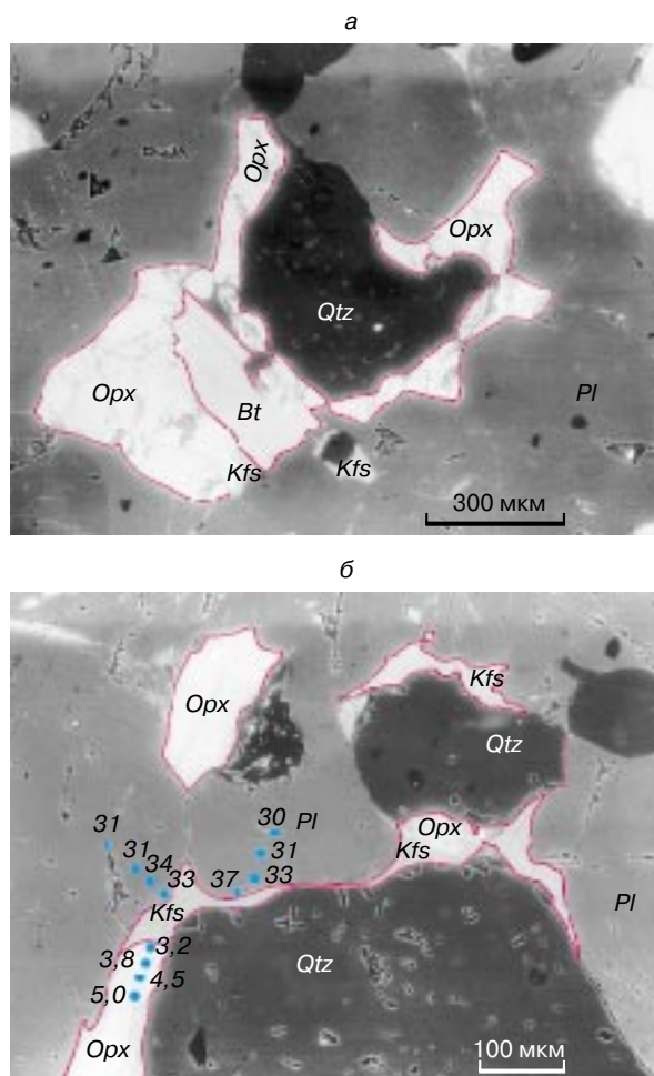
Рис. 3. Реакционная кайма Opx и Kfs , возникшая на границе зерен биотита и кварца (а), и развитие реакционной каймы Kfs (б) в гиперстенсодержащем гнейсе из комплекса Сулкава, в Южной Финляндии, при T = 720 \pm 30^\circ C , P = 6,2 \pm 0,4 кбар, a_{H_2O} = 0,4 \pm 0,03 . Цифры на микрофотографии (б) обозначают содержание анортитового (кальциевого) компонента в плагиоклазе ( Pl ) и содержание Al_2O_3 в ортопироксене ( Opx )
