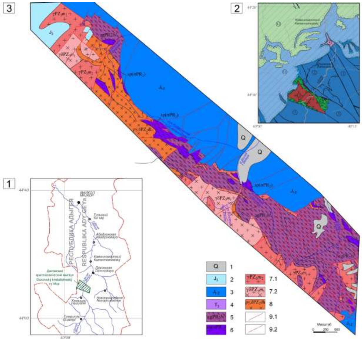
Рис. 1. Положение и геологическое строение территории: 1 – положение Даховского поднятия; 2 – тектоническая схема (геологические структуры, обозначенные на схеме: 1 – Северо-Кавказская моноклираль: 1.1. – область развития келловей – верхнеюрских пород, 1.2. – область развития меловых пород; 2–7 – Лабино-Малкинская зона прерывистой складчатости: 2 – Догуакская покровно-складчатая зона ( J_{1-2} ), 3 – Сахрайская зона сдвигово-надвиговых дислокаций ( J_{1-2} ), 4 – Руфабгинский выступ (гранитоидный массив - PZ_{2-3} ; осадочный комплекс - T ); 5 – Даховская антиклиналь ( J_{1-2} ); 6 – Даховский выступ: 6.1 – гранитоидный массив ( PZ_{2-3} ), 6.2. – метаморфическая толща балканского комплекса ( PR_{2?} ), 6.3 – серпентиниты апогипербазитовые ( PR_{2?} ); 7 – Дудугушская синклиналь( J_{1-2} )); 3 – геологическая карта северного фланга Даховского поднятия (по Менькову В.М., Качурину В.Ф. (1964 г.) с дополнениями): 1 – четвертичные образования, 2 – келловей – кимериджский осадочный комплекс (известняки, доломиты, песчаники, гравелиты, конгломераты); 3 – нижне – среднеюрский осадочный комплекс (аргиллиты, алевролиты, песчаники), 4 – верхнетриасовый комплекс (известняки, песчаники), 5 – балканский метаморфический комплекс (амфиболиты, амфиболовые гнейсы), 6 – серпентиниты апогипербазитовые беденского комплекса, 7.1 – малкинский гранитоидный комплекс (граниты), 7.1 – малкинский гранитоидный комплекс (гранодиориты), 8 – даховский гранитоидный комплекс (плагииграниты, диориты), 9 – разломы прослеженные, 9.2 – разломы предполагаемые. /
