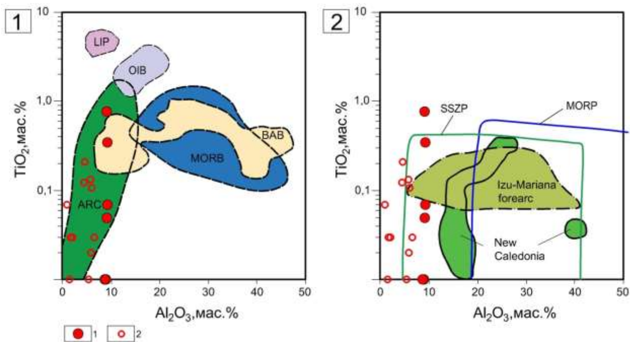
Рис. 5. Положение составов хромшпинелидов (внутренние области) относительно полей составов типичных геодинамических обстановок (по Ghazi et al., 2011; Kamenetsky, Crawford, Meffre, 2001; Rollinson, Adetunji, 2015): LIP – базальты крупных изверженных провинций; OIB – базальты океанических островов; ARC – островодужные базальты; BAB – базальты задуговых бассейнов; MORB – базальты срединно-океанических хребтов; SSZP – океанические надсубдукционные перидотиты. Составы внутренних частей хромшпинелидов серпентинитов Даховского поднятия: 1 – исходные; 2 – измененные части зерен.
