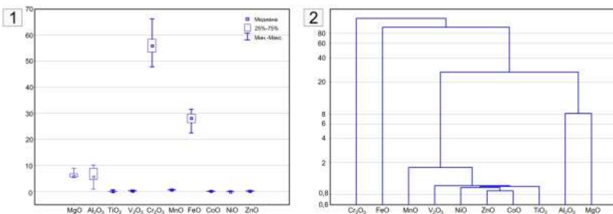
Рис. 3. Результаты статистической обработки данных элементного анализа хромшпинелидов: 1 – основные описательные статистики; 2 – дендрограмма (метод одиночной связи; указаны евклидовы расстояния, шкала логарифмическая).
