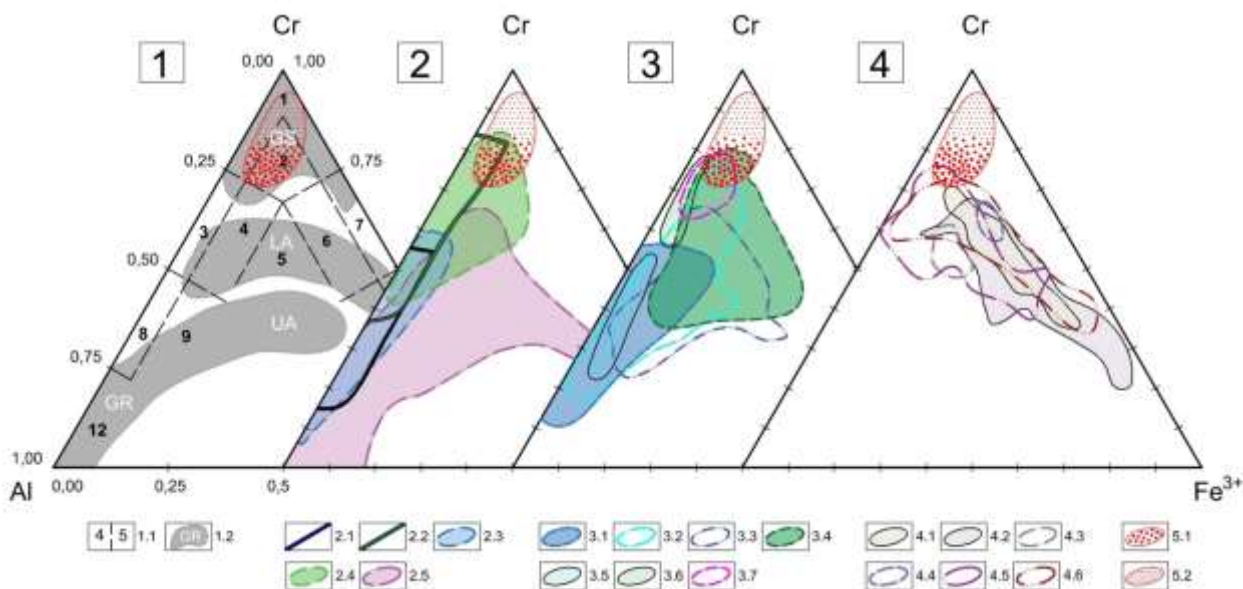
Рис. 4. Положение составов хромшпинелидов (внутренние области) на диаграммах Al - Cr - Fe 3+ :
